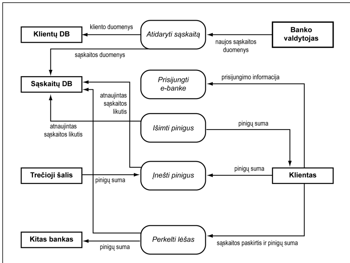
III-3 pav. Detalus duomenų srautų modelis
