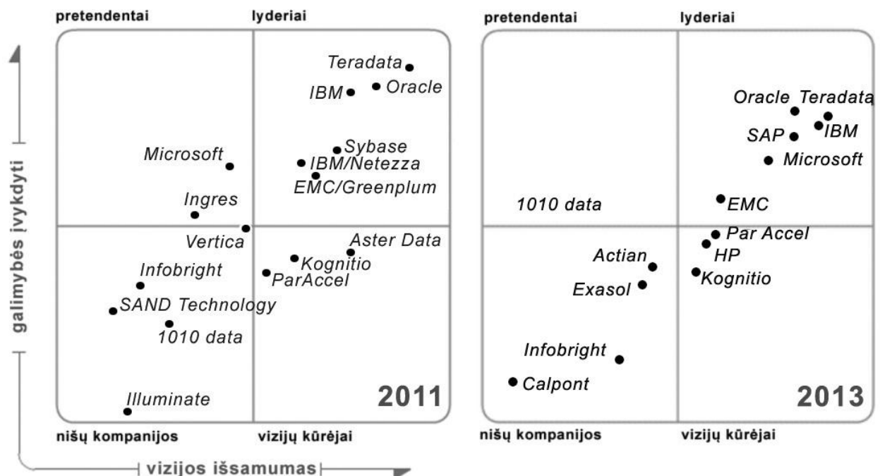
I-3 pav. Duomenų saugyklų DBVS „magiškas kvadratas“ 1 .
