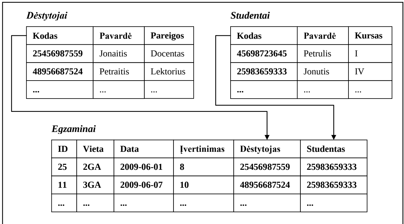
IV-13 pav. Ryšių vaizdavimas lentelių modelyje.
